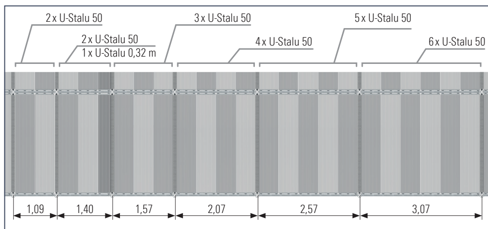
Stalu U-vlonder 50 in Allround ruimtesteiger
