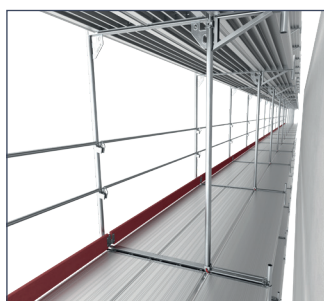
Stalu U-vlonder 50 met console 0,50 m
