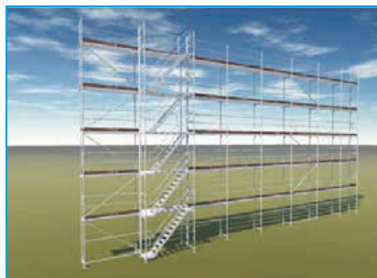
3D-presentatie gevelsteiger met steigerbordestrappen gecreëerd met LayPLAN CLASSIC.
