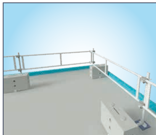
Compacte plat dakrandbeveiliging gemonteerd met rolsteigerleuningingen.
